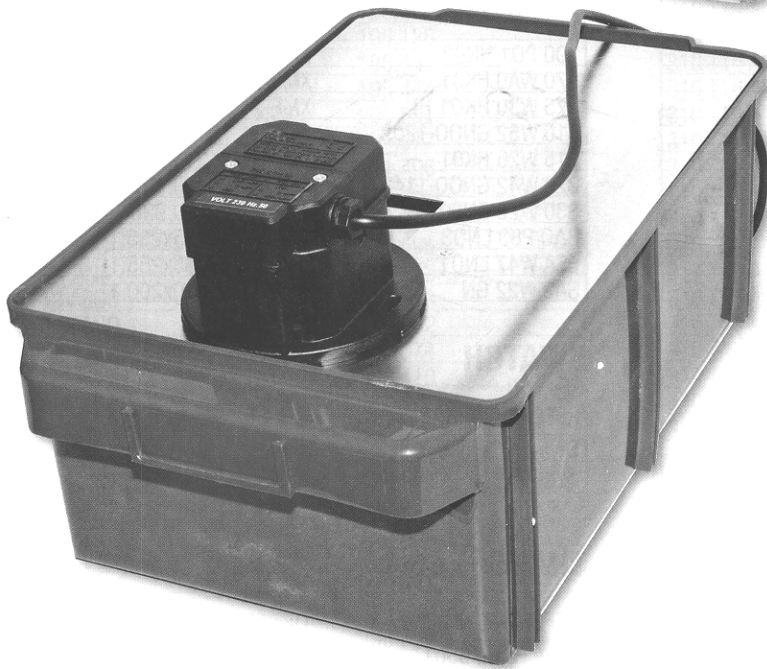
Nr. 16 Kronoglas- Maschine mit Getriebemotor zum Schleifen von Mineralgläsern
