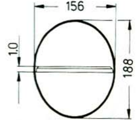
Pl. E 188×156
