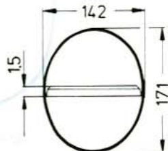
Pl. E 171 × 142
