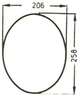
E 258×206.1 Konkav
