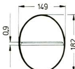
Pl. E 182 × 149
