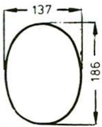
E 186×137.1 Konkav
